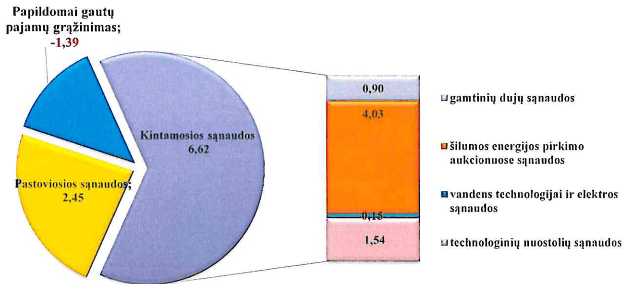
4 paveikslas. 2024 m. kovo mėn. šilumos kainos dedamosios, 7,68 ct/kWh (be PVM)
